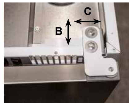
Övre gångjärn, bild 1
